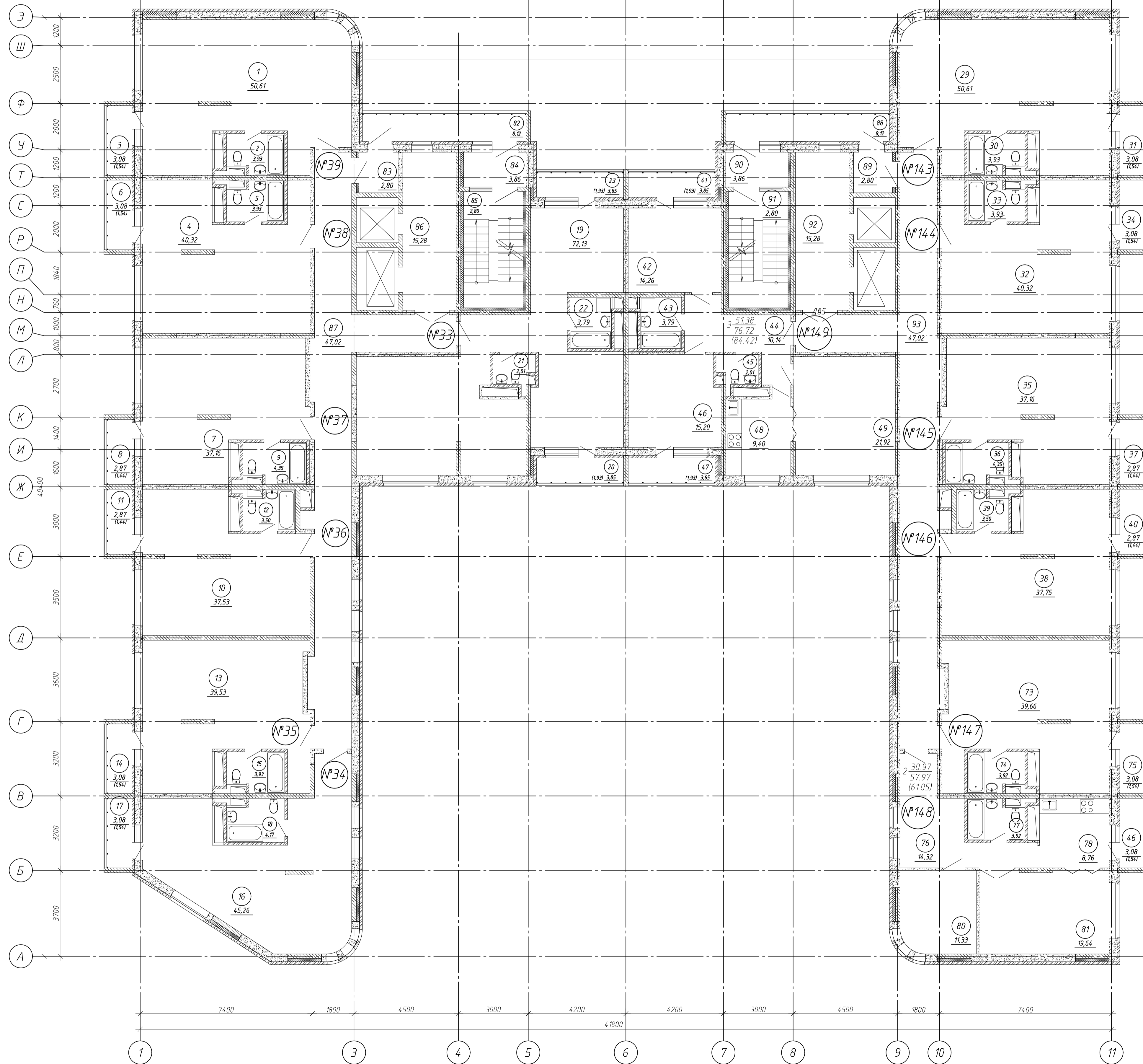
План шестого этажа
